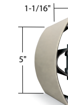
SCR-50N shown
